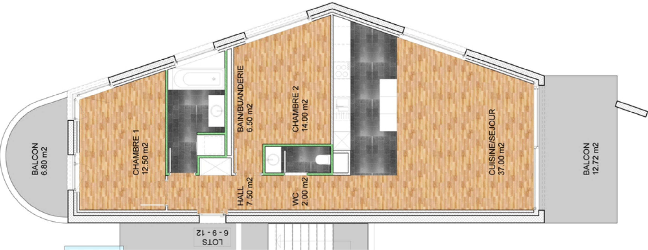
PLAN APPARTEMENT TYPE 3.5 Pièces, ech. 1/100e
